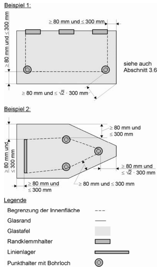
Bild 1: Prinzipskizze Glasauskragung
